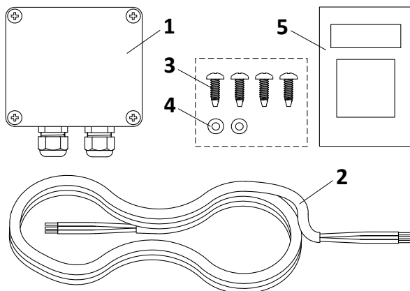
Рис. 1 – Комплект поставки
