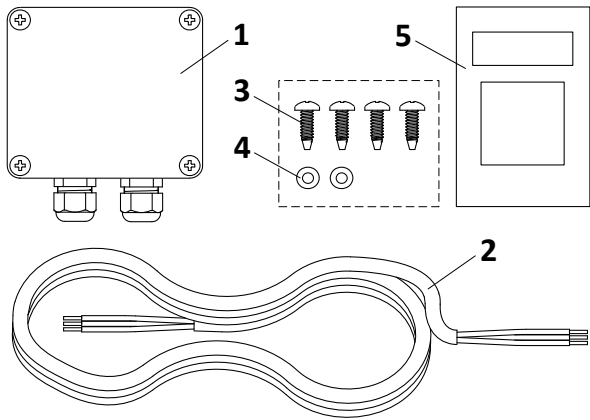
Abbildung 1 – Lieferumfang
