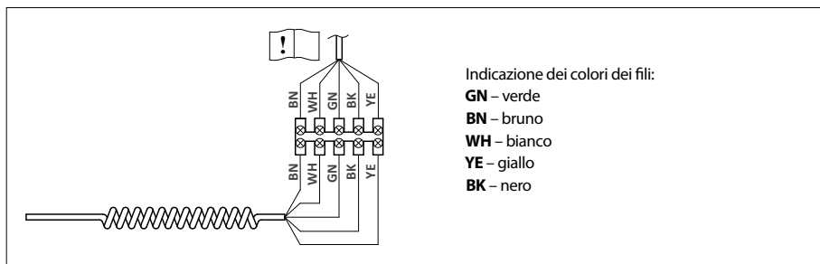
Figura 2 – Montaggio
