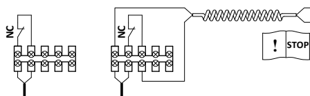
Figura 2 – Montaggio
