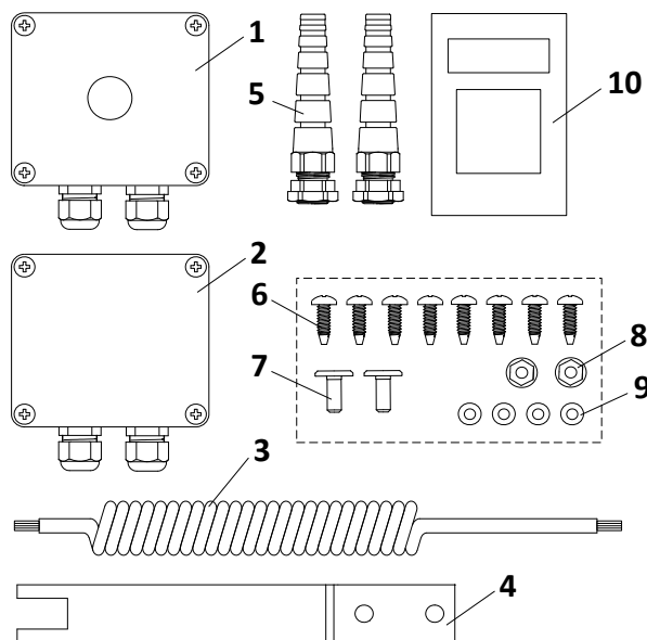
Рис. 1. Комплект поставки
