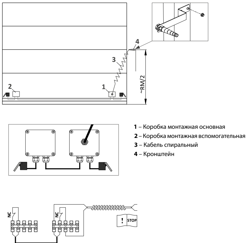
Рисунок 2 – Монтаж
